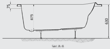
Sec A-A
