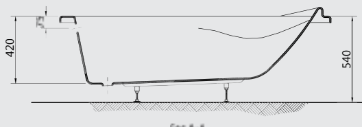
Side A-B
