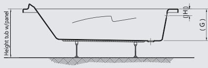
Sec A-A
