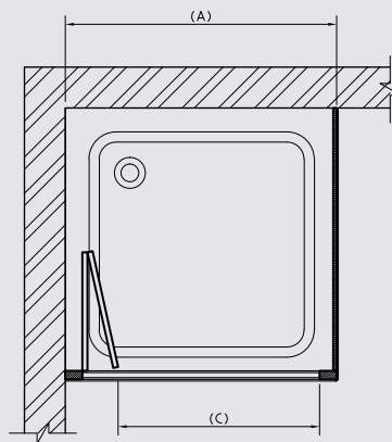
Sec. A-A
