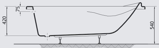
Sec A-A
