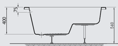
Sec A-A
