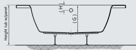
Sec A-A
