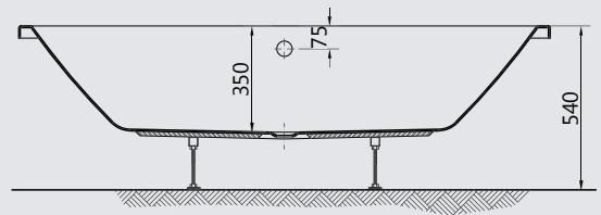
Sec A-A
